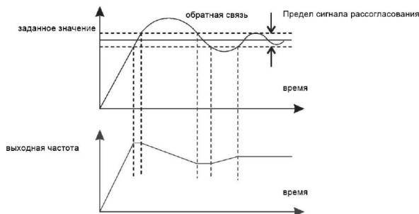
Рис. 6.24 — Отклонение ПИД-управления
