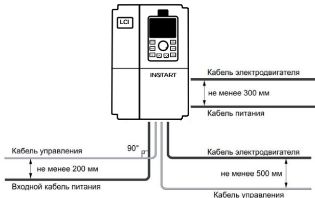
Рис. 3.7 – Графическое представление расстояний между кабелями
