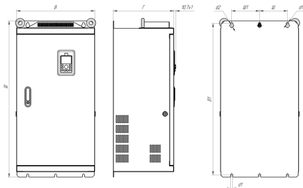
Рис. 2.6 — Габаритные и установочные размеры устройств серии LCI в металлическом корпусе
