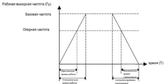
Рис. 6.1 - Время разгона/торможения
